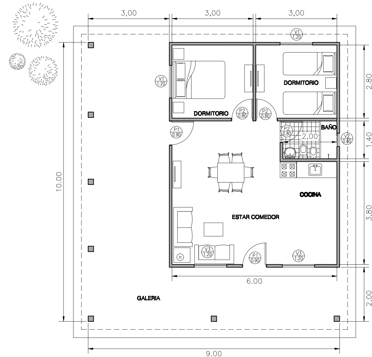
PLANTA
