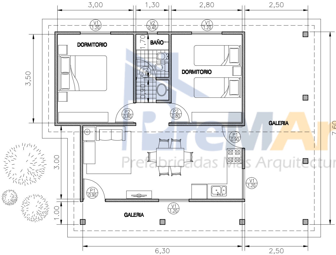
PLANTA CABAÑA
